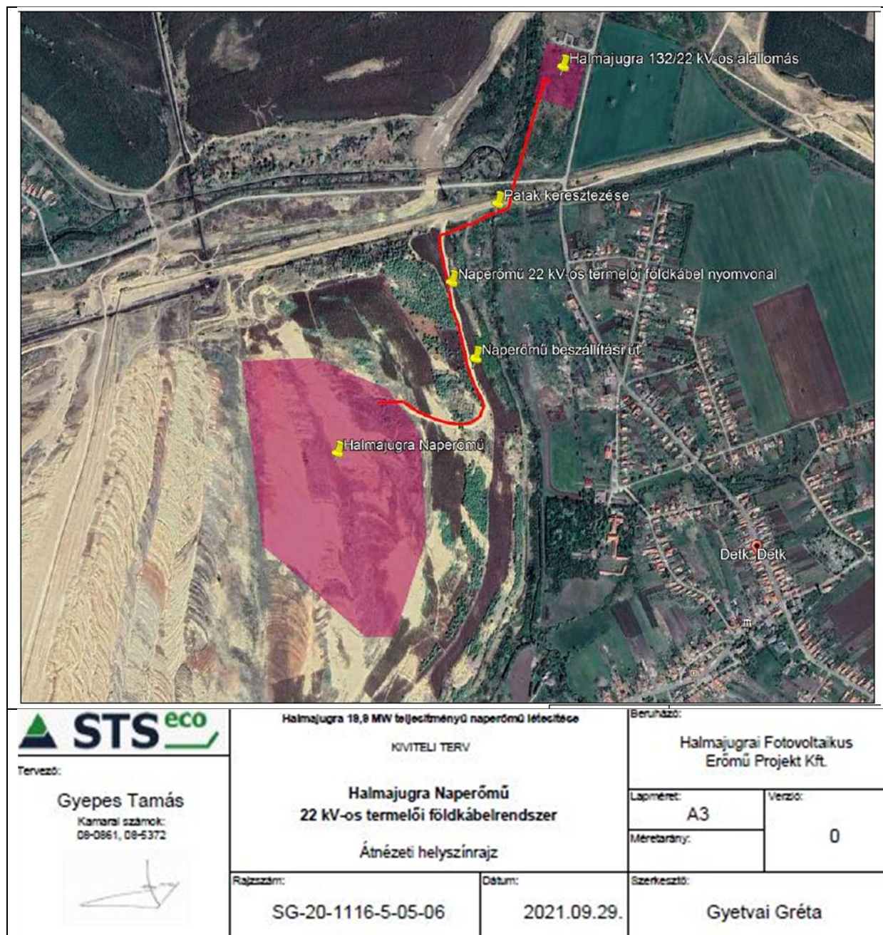
2. ábra: Átnézeti helyszínrajz a teljes projektről (forrás: (forrás: Halmajugra 19,9 MW teljesítményű naperőmű létesítése, Kiviteli terv, STS ECO, 2021.szeptember)
