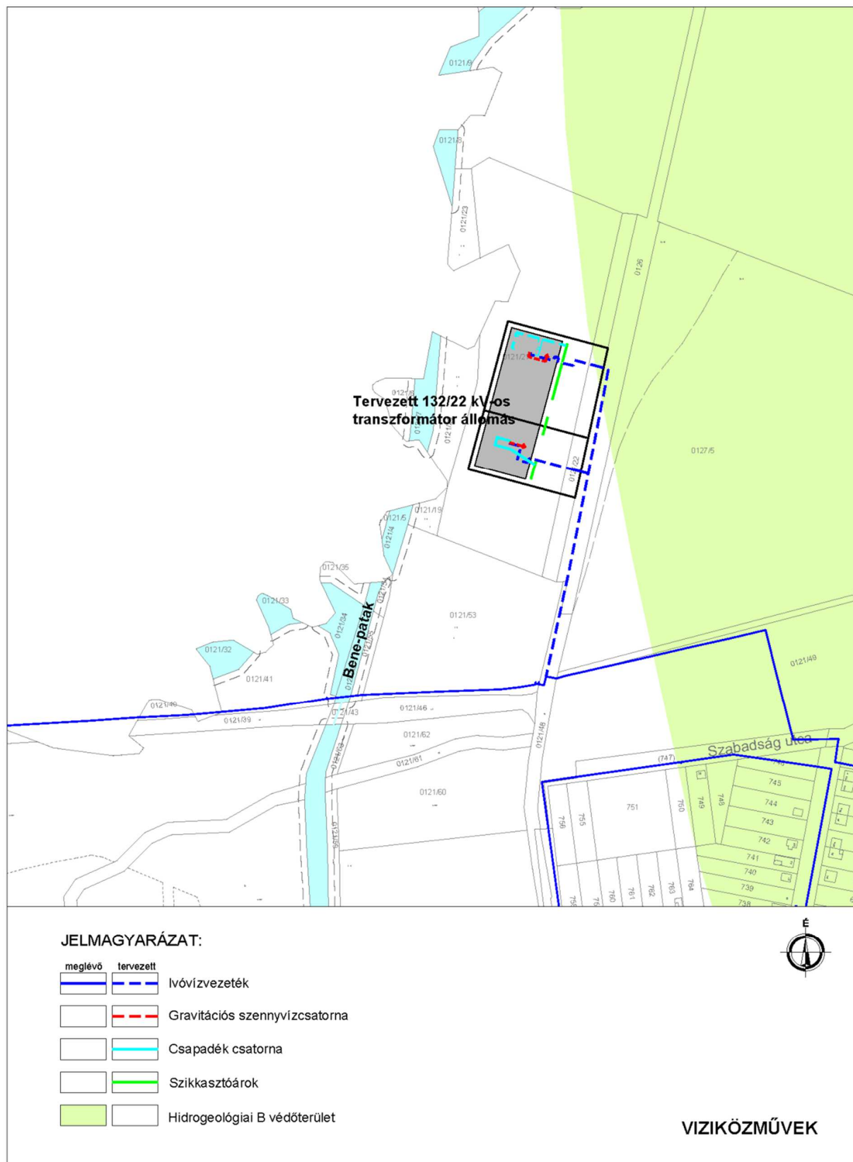
6. ábra: Viziközművek (készítette: KÉSZ Közmű Kft.)
