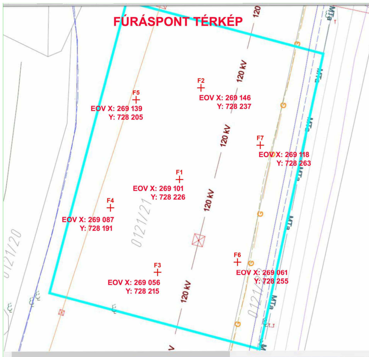
8. ábra: A feltáró fúrások helye EOVS koordinátákkal
