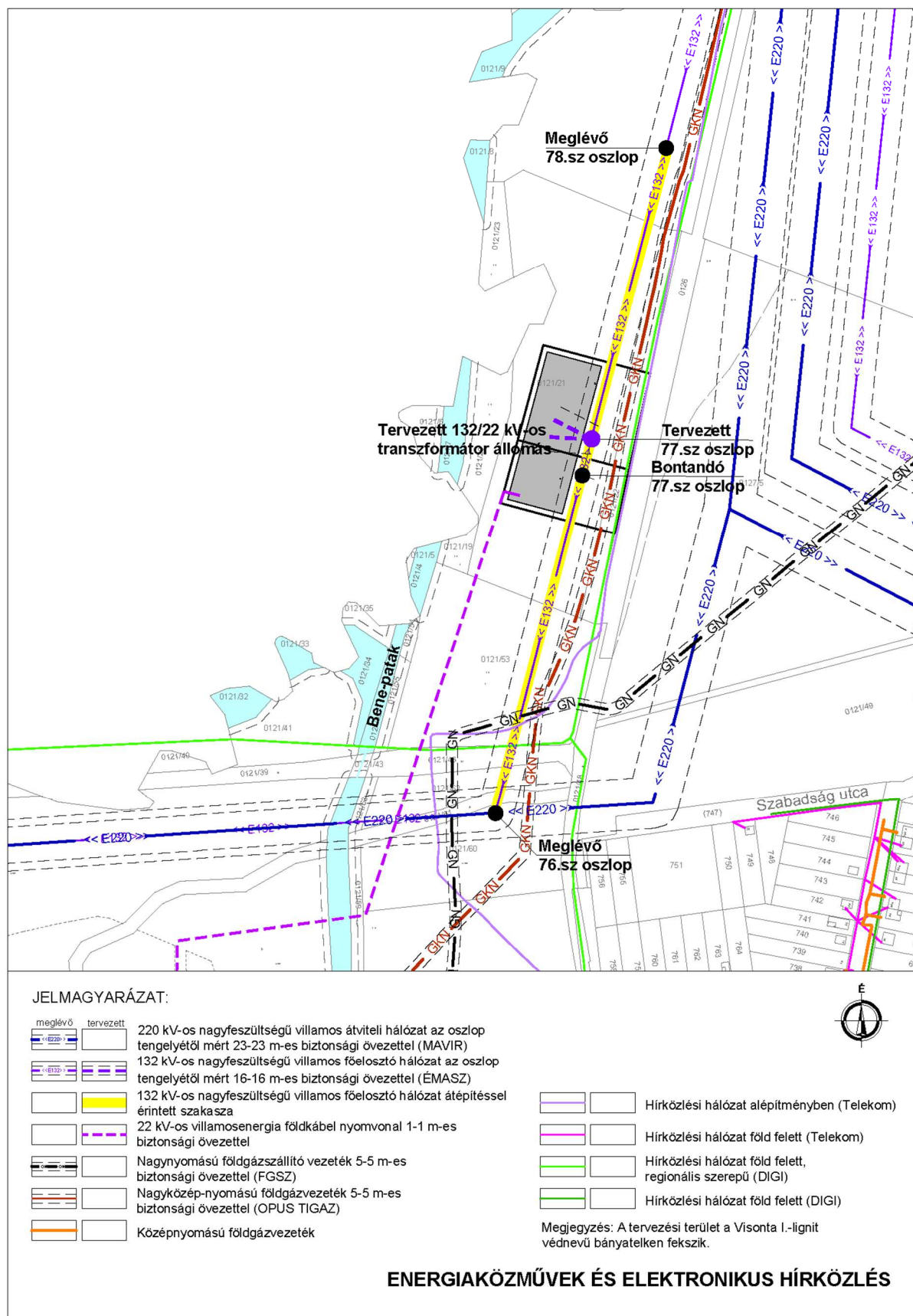
7. ábra: Energiaközművek és elektronikus hírközlés (készítette: KÉSZ Kft.)
